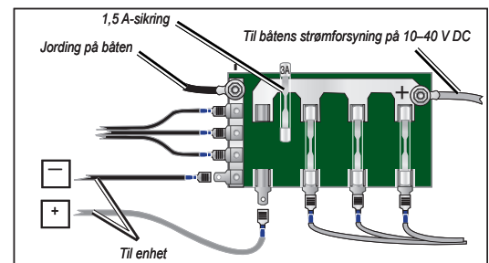
Eksempel på sikringsblokk
